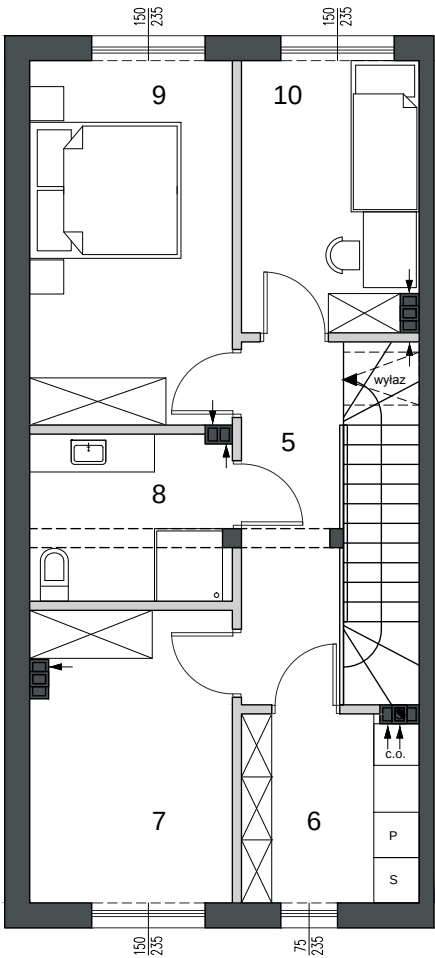
rzut piętra
