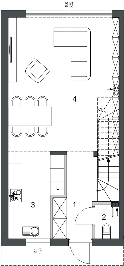
rzut parteru
